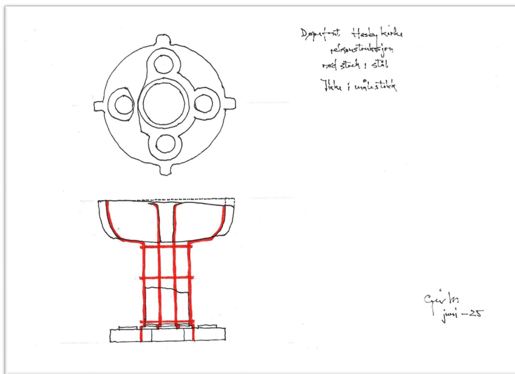
Figur 3: Et foreløpig utkast til hvordan stativet kan komme til å utformes.
